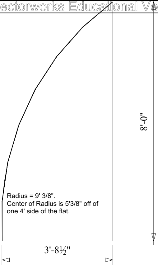
2 Front Scale: 1/2" = 1'-0"
